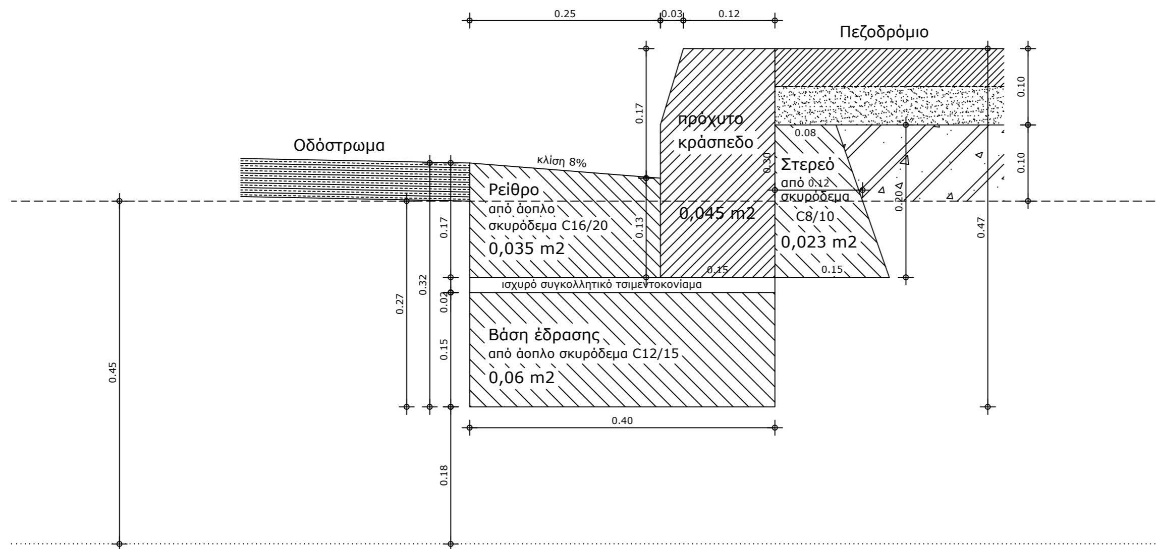
ΤΥΠΙΚΗ ΔΙΑΤΟΜΗ ΚΡΑΣΠΕΔΟΡΕΙΘΡΩΝ ΕΚ ΠΡΟΚΑΤΑΣΚΕΥΑΣΜΕΝΩΝ ΚΡΑΣΠΕΔΩΝ
